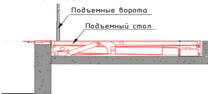
Пример установки докового стола
